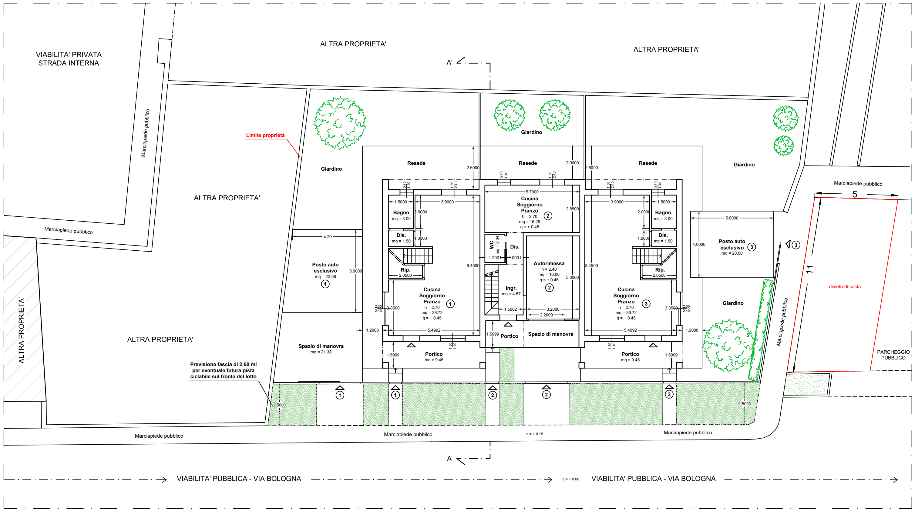
PLANIMETRIA GENERALE PIANO TERRA SCALA 1:100
