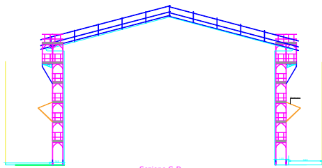
Sezione C-D
