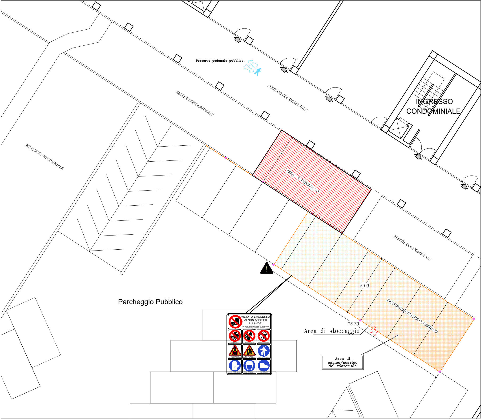
PLANIMETRIA GENERALE
