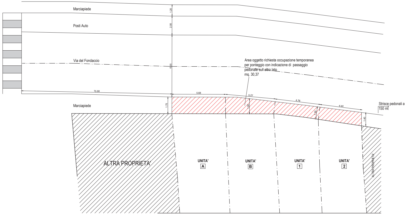
PLANIMETRIA
