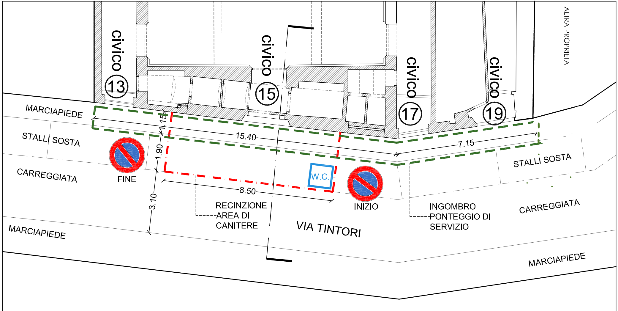
PLANIMETRIA AREA DI CANTIERE ESTERNA
